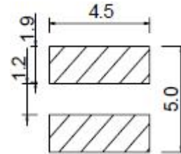
LAND PATTERNS(mm) 焊盘尺寸
