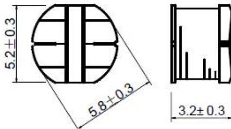
DIMENSIONS(mm) 外型尺寸
