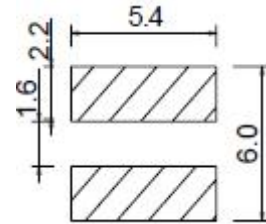
LAND PATTERNS(mm) 焊盘尺寸
