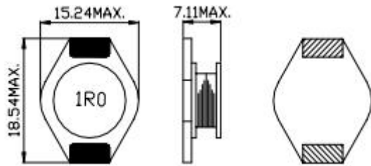
DIMENSIONS(mm) 外型尺寸
