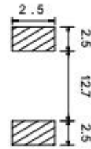
LAND PATTERNS(mm) 焊盘尺寸
