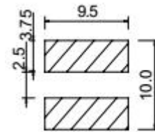
LAND PATTERNS(mm) 焊盘尺寸
