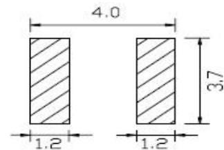
LAND PATTERNS(mm) 焊盘尺寸
