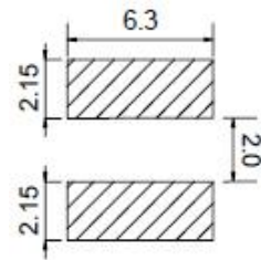
LAND PATTERNS(mm) 焊盘尺寸
