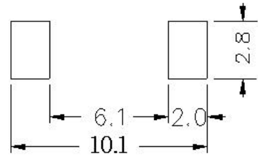
LAND PATTERNS(mm) 焊盘尺寸
