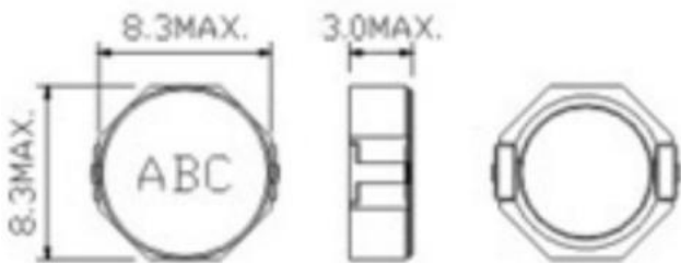
DIMENSIONS(mm) 外型尺寸
