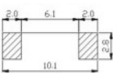
LAND PATTERNS(mm) 焊盘尺寸
