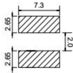
LAND PATTERNS(mm) 焊盘尺寸
