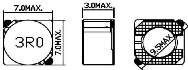
DIMENSIONS(mm) 外型尺寸
