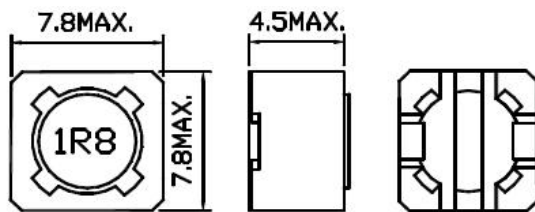
DIMENSIONS(mm) 外型尺寸
