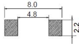
LAND PATTERNS(mm) 焊盘尺寸
