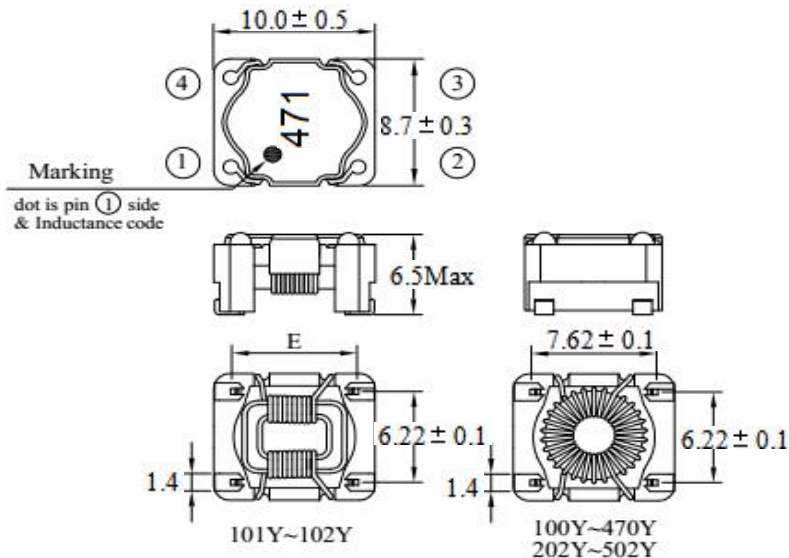
DIMENSIONS(mm) 外型尺寸
