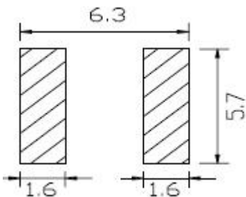
LAND PATTERNS(mm) 焊盘尺寸
