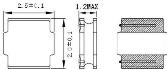
DIMENSIONS(mm) 外型尺寸
