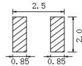
LAND PATTERNS(mm) 焊盘尺寸
