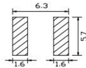
LAND PATTERNS(mm) 焊盘尺寸
