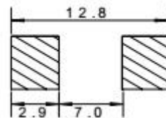
LAND PATTERNS(mm) 焊盘尺寸
