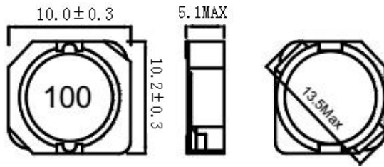
DIMENSIONS(mm) 外型尺寸
